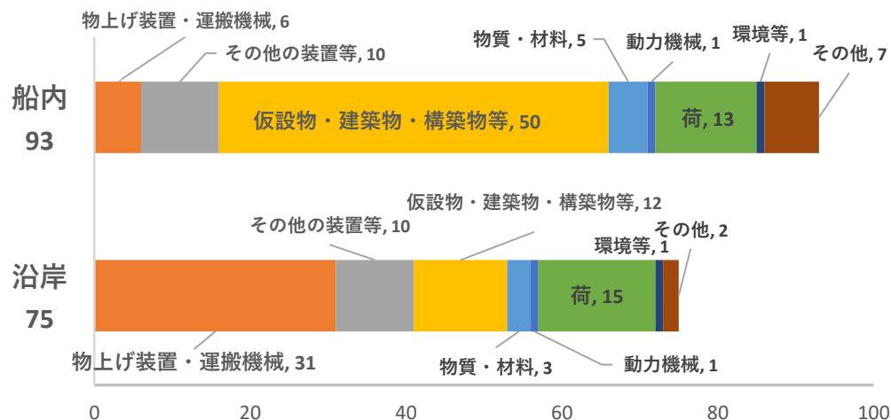
(第2図) 墜落・転落災害の起因物別発生件数(平成30年～令和4年)
